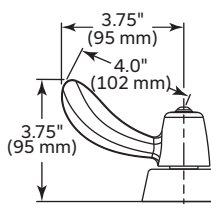
Handle 2 Poignée 2 Manija 2
