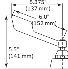
Handle 5 Poignée 5 Manija 5
