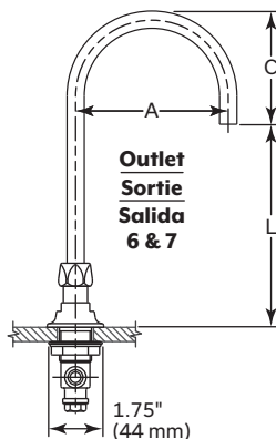
Gooseneck Spouts Bec col de cygne Salida de agua en pico
