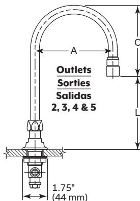
Gooseneck Spouts Bec col de cygne Salida de agua en pico
