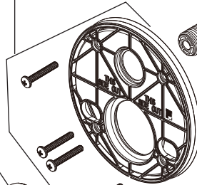
RP100386▲ Valve Seal Sello de la válvula Garniture d'étanchéité
