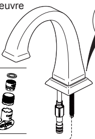
RP91142-1.2 1.2 GPM (4.5 L/min) Aerator & Wrench Aireador y Llave Aérateur et Clé
