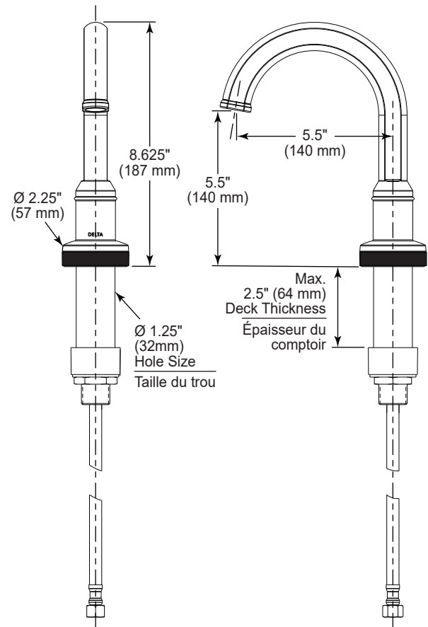
Single Hole Faucet with Black Spacer Robinet monotrou avec cale d'espacement noire
