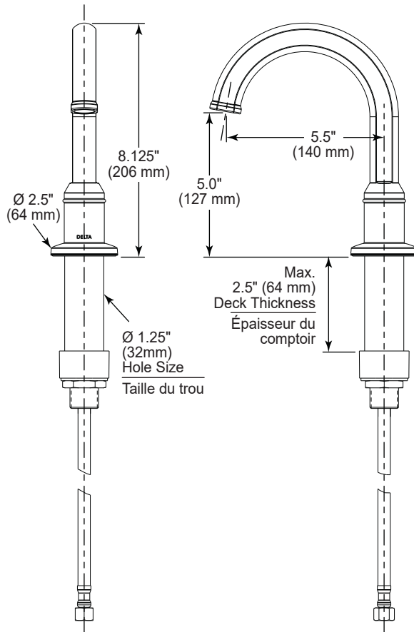
Single Hole Faucet without Black Spacer Robinet monotrou sans cale d'espacement noire
