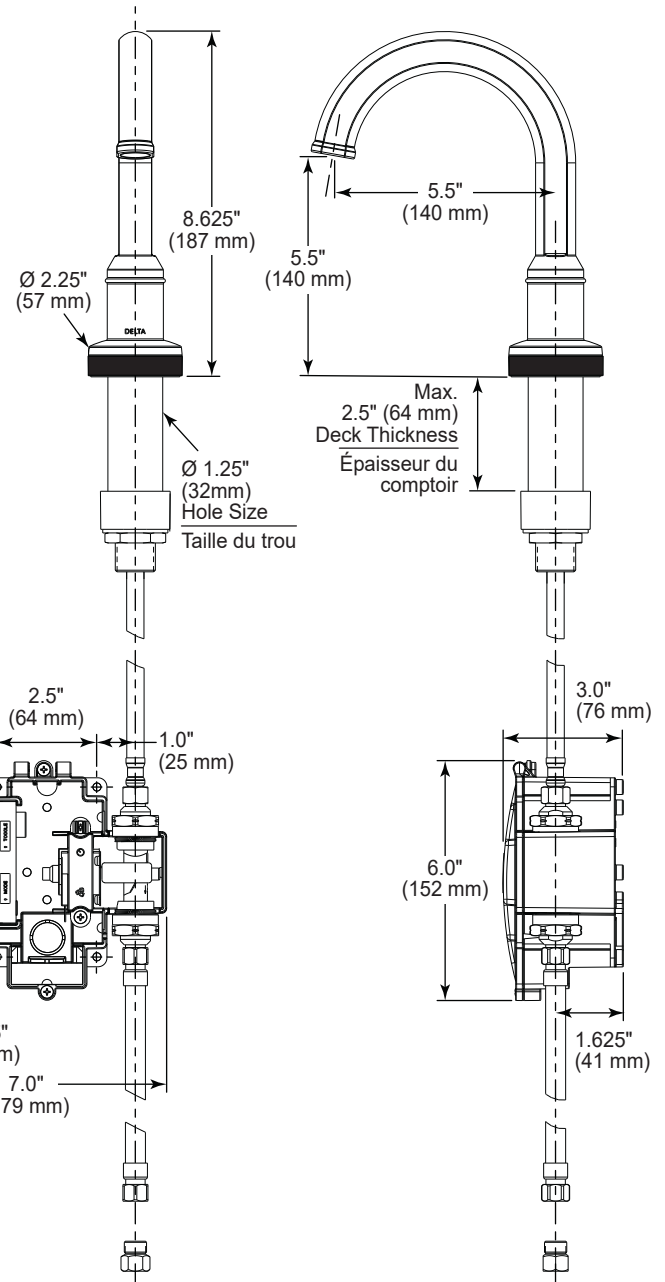
Single Hole Faucet with Black Spacer Robinet monotrou avec cale d'espacement noire
