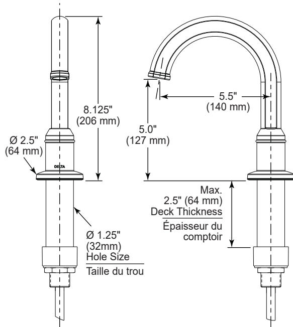
Single Hole Faucet without Black Spacer Robinet monotrou sans cale d'espacement noire
