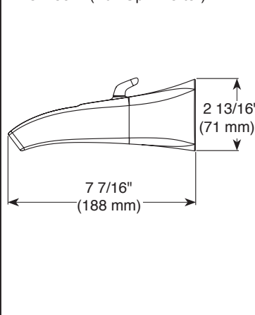
RP82490 ▲ (Pull-Up Diverter)
